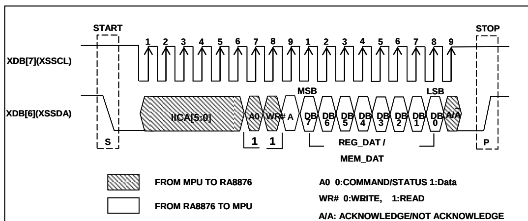
圖 7-21 : Data Read on IIC-Bus
