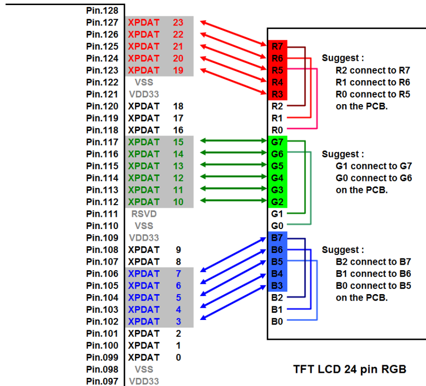
Figure 10-3 : RA8876 色深 16bit 脚位与 LCD 屏幕脚位对应
