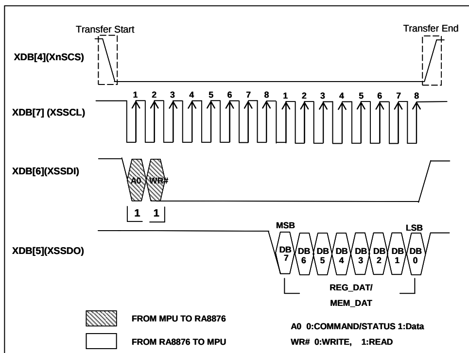
圖 7-15 : Data Read on 4-Wire SPI-Bus
