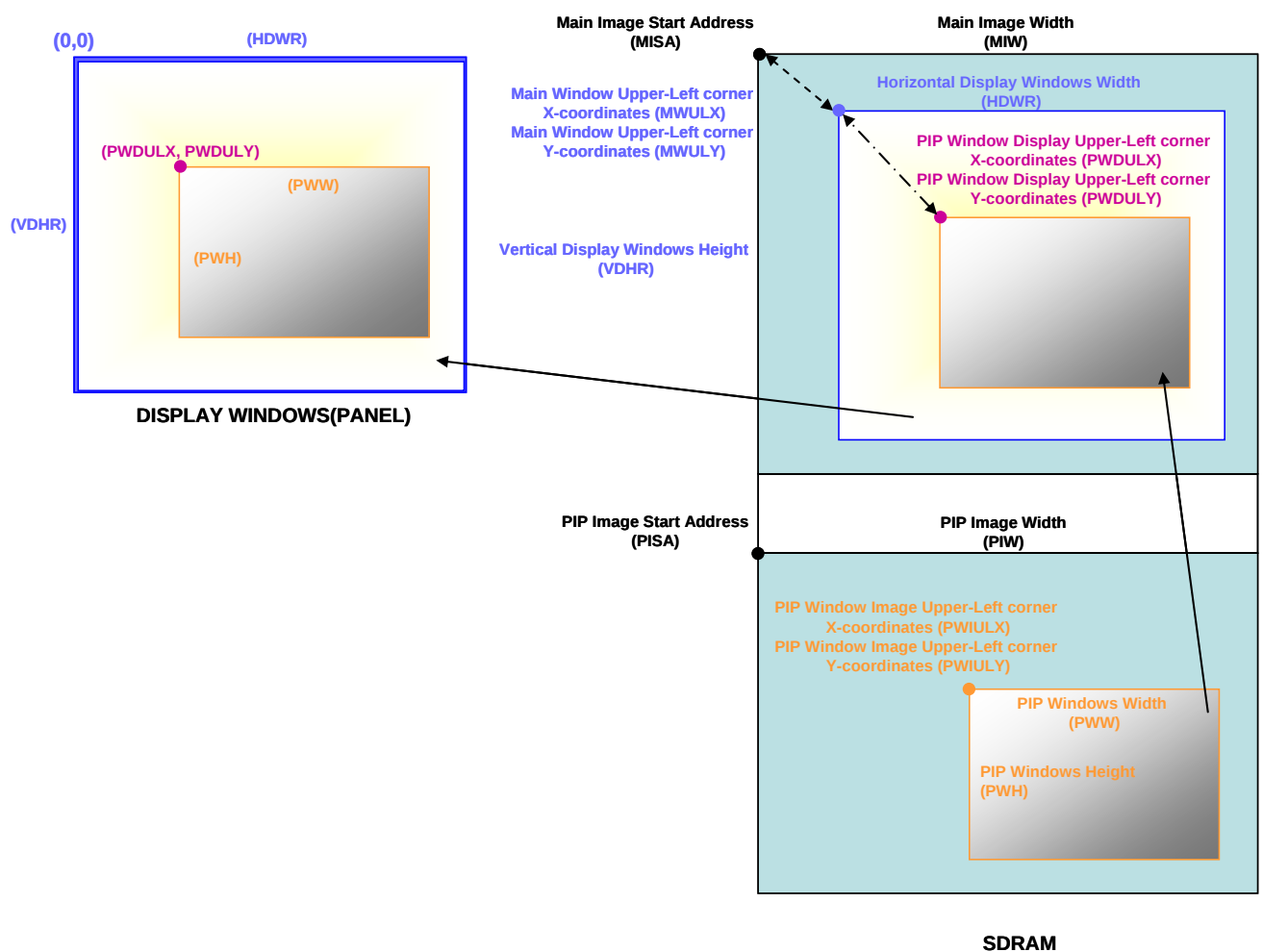
圖 19-2 LCD Display
