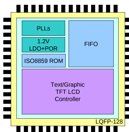
圖 1-2 : Chip Diagram
