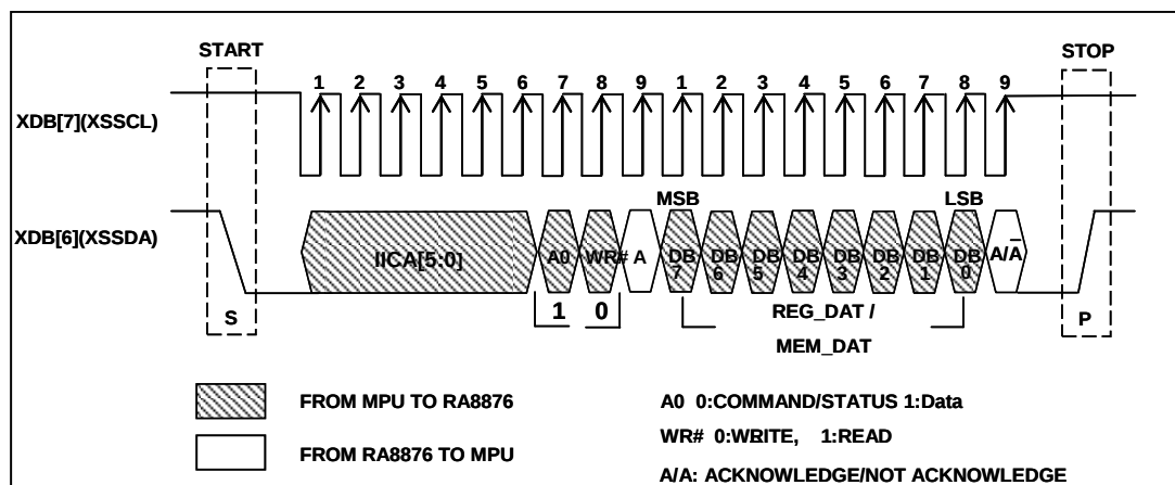
圖 7-20 : Data Write on IIC-Bus
