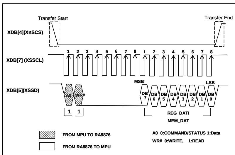
圖 7-10 : Data Read on 3-Wire SPI-Bus
