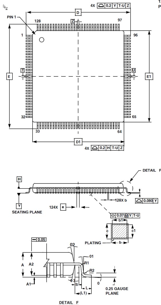
圖 3-2 : RA8876 Package Outline Dimensions
