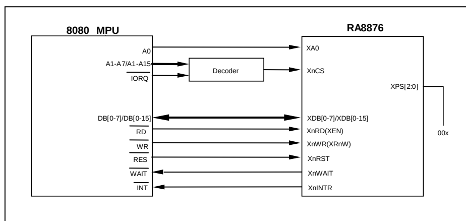
圖 7-1 : 8080 MPU Interface
