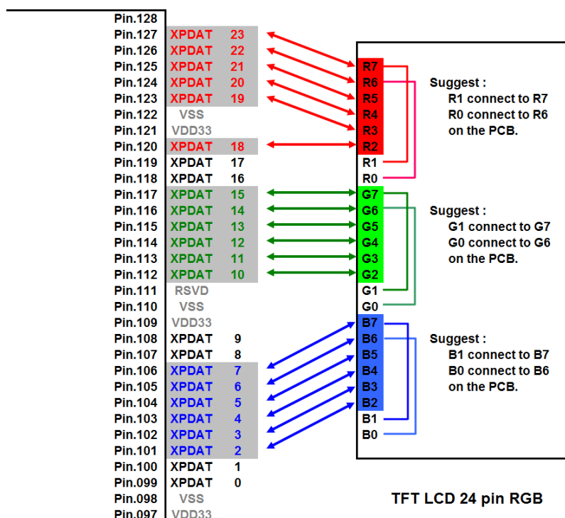
Figure 10-2 : RA8876 色深 18bit 脚位與 LCD 螢幕脚位對應
