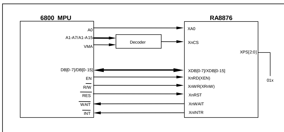
圖 7-2 : 6800 MPU Interface
