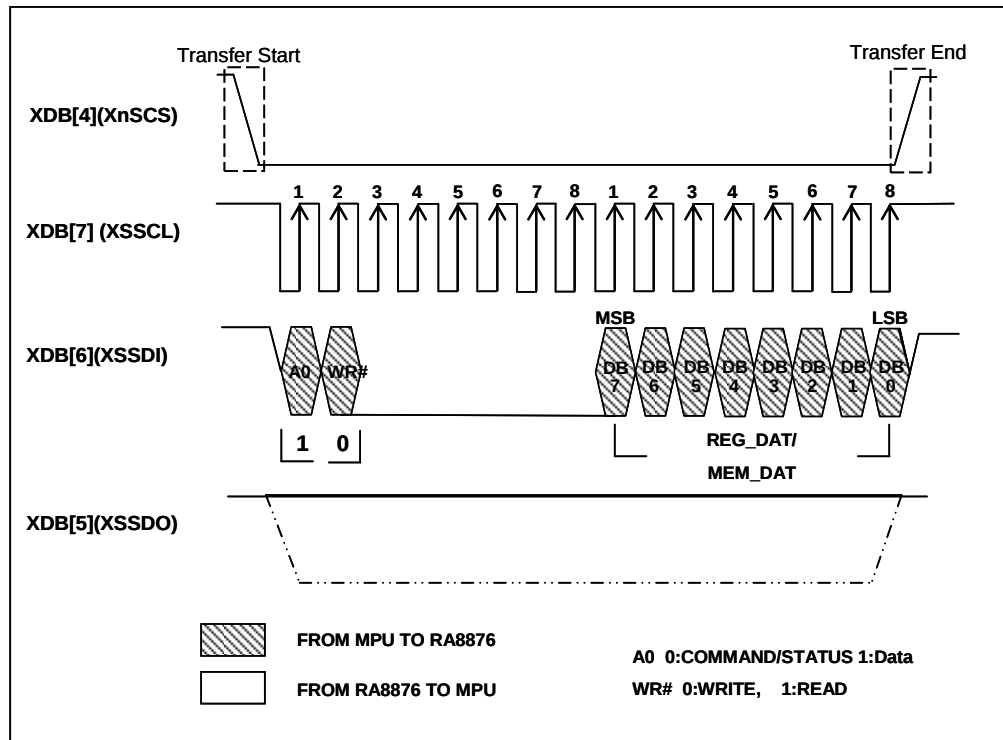
圖 7-14 : Data Write on 4-Wire SPI-Bus
