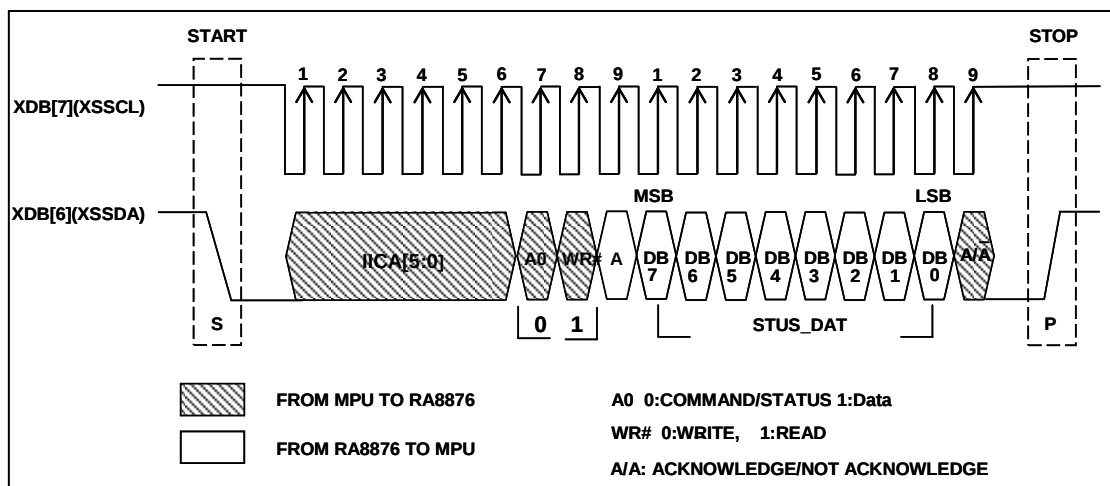
圖 7-23 : Status Read on IIC-Bus
