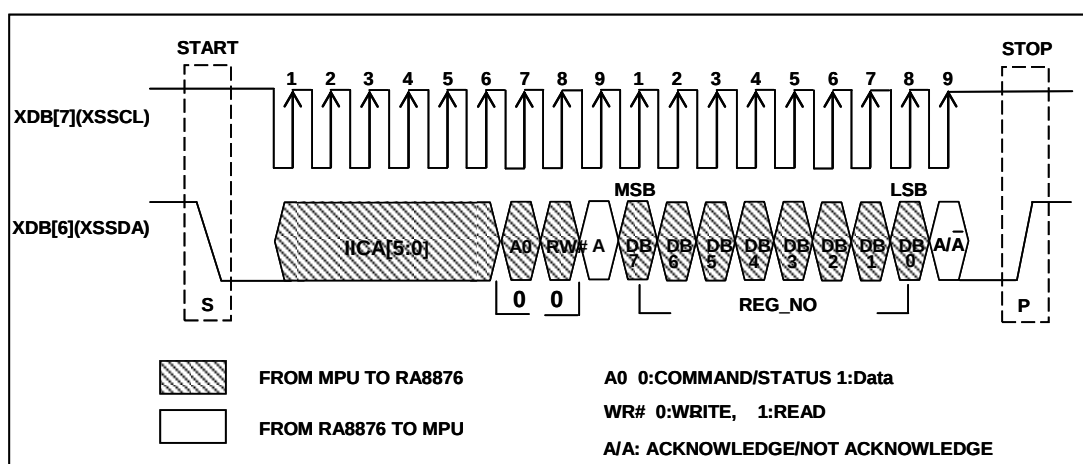
圖 7-22 : CMD Write on IIC-Bus
