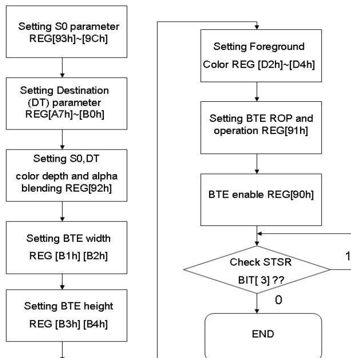
圖 13-38 : Flow Chart
