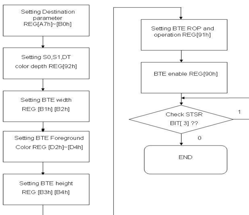
圖 13-40 : Flow Chart
