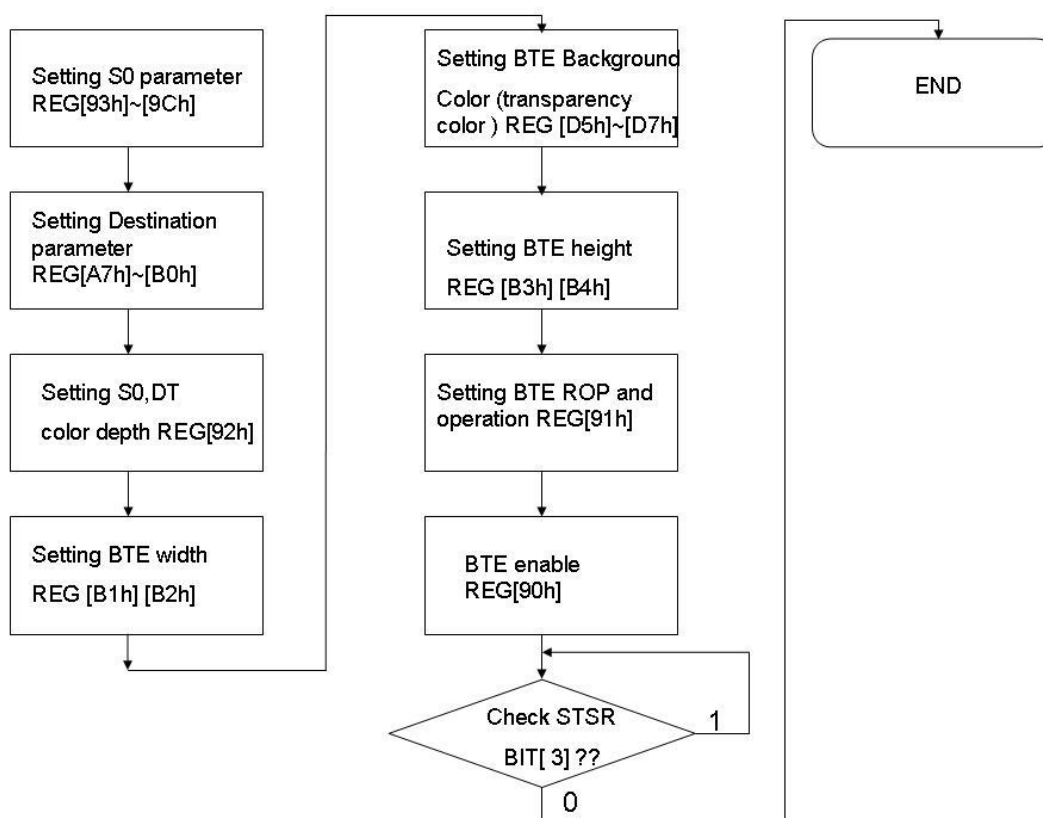
圖 13-12 : Flow Chart
