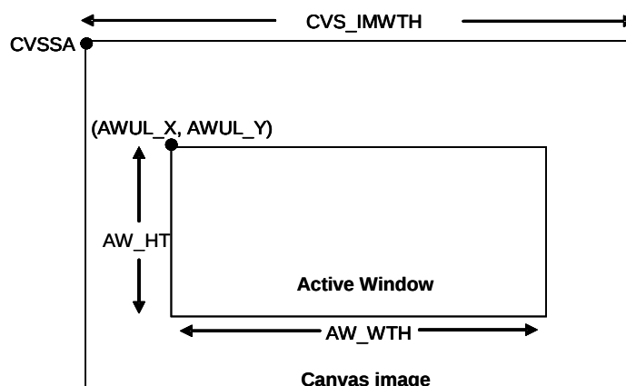
圖 19-4 : Active Window
