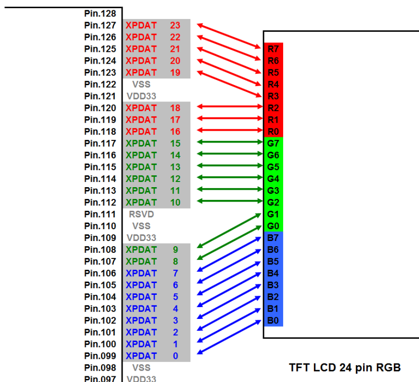
Figure 10-1 : RA8876 色深 24bit 脚位与 LCD 屏幕脚位对应
