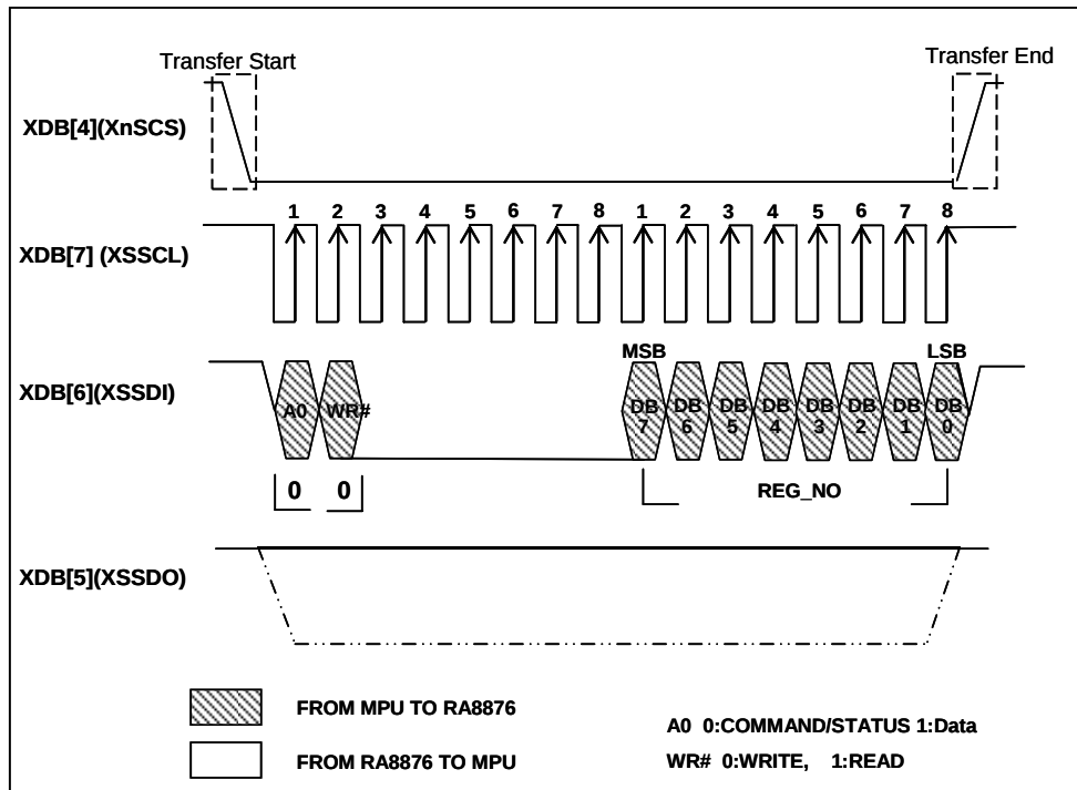
圖 7-16 : CMD Write on 4-Wire SPI-Bus
