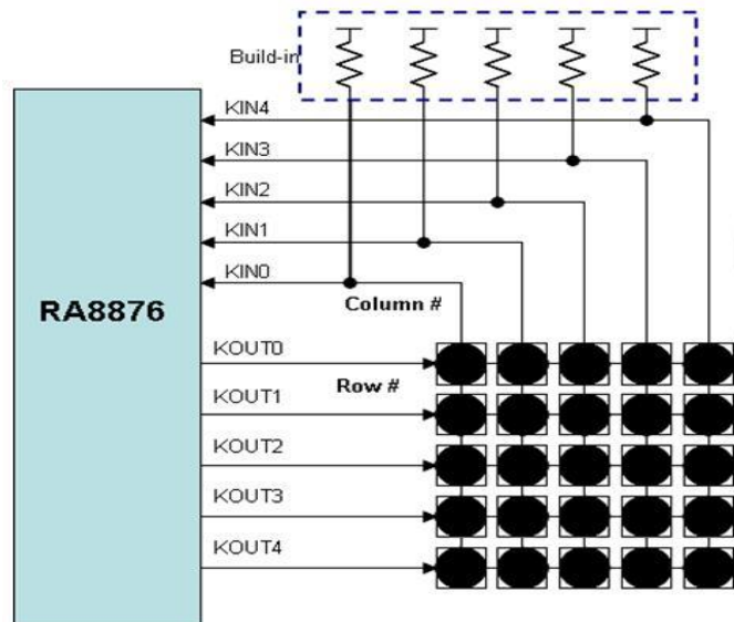
圖 17-1 : Key-Pad Application
