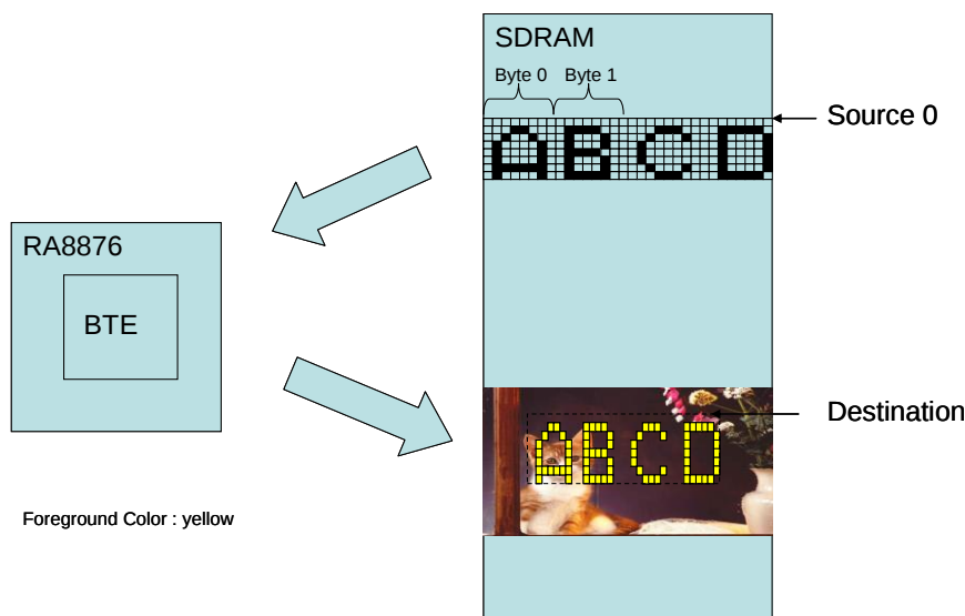
圖 13-37 : Hardware Data Flow
