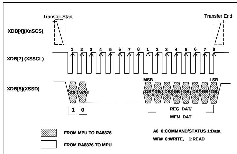
圖 7-11 : Date Write on 3-Wire SPI-Bus
