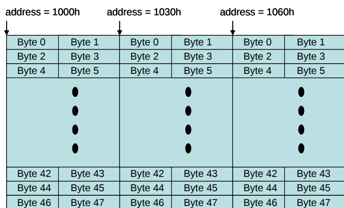
圖 14-6 : Font Array 12x24 in SDRAM
